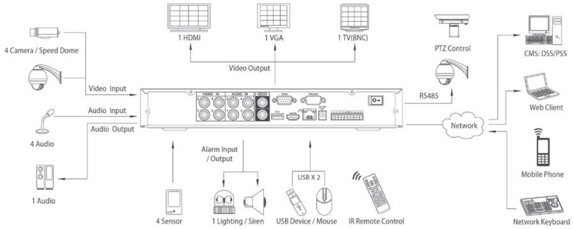
DSS-DVR0404H
